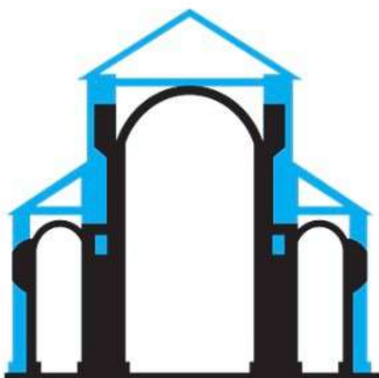
Схема романского храма в разрезе
