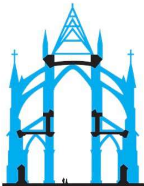
Схема готического храма в разрезе
