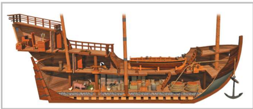
Каравелла. Внутреннее устройство. Современная реконструкция
