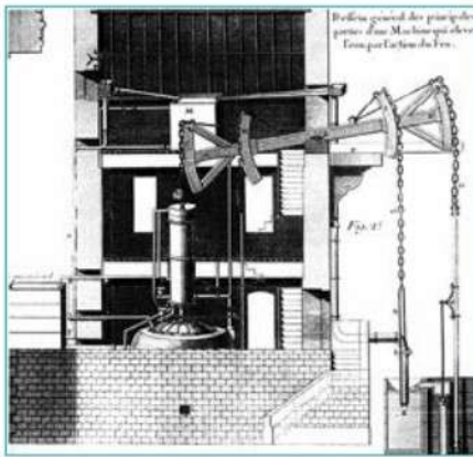
Паровая машина Ньюкомена. Гравюра из книги Б. Белидора «Гидравлическая архитектура». XVIII в.
