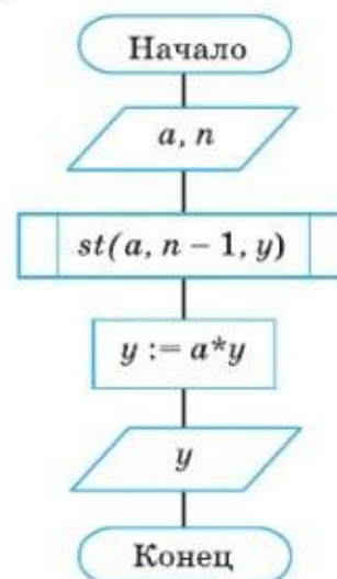
Рис. 1.6. Рекурсивный алгоритм возведения в степень
