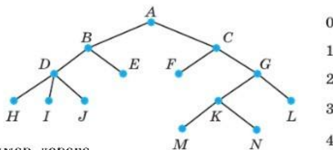
Рис. 2.16. Пример дерева
