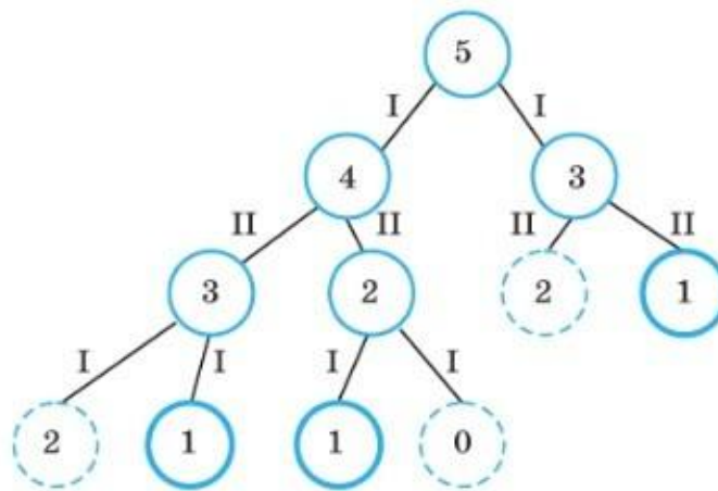
Рис. 2.18. Дерево игры
