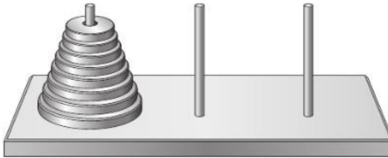
Рис. 1.7. Головоломка «Ханойская башня»
