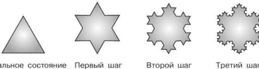
Рис. 1.8. Шаги алгоритма построения снежинки Коха
