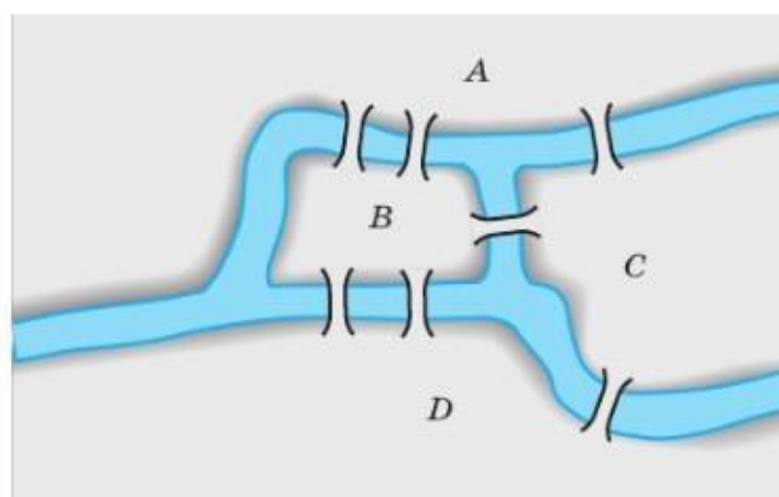
Рис. 2.11. Мосты Кёнигсберга
