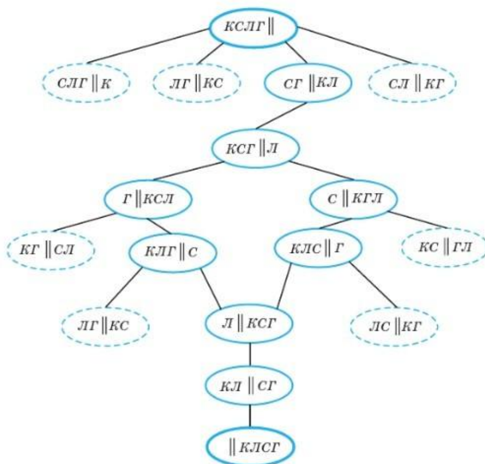
Рис. 2.15. Граф переправы
