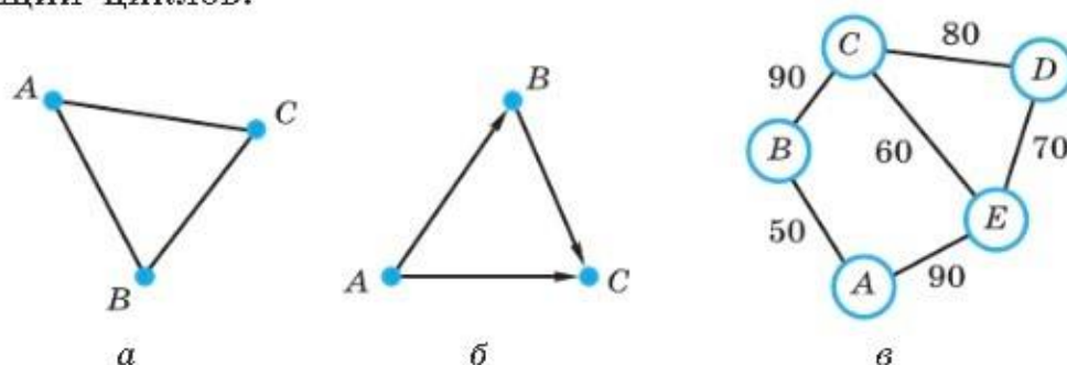
Рис. 2.10. Графы
