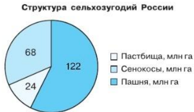
Рис. 3.12. Пример круговой диаграммы
