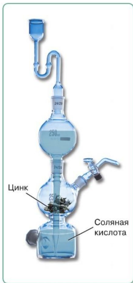
Рис. 35. Аппарат Киппа
