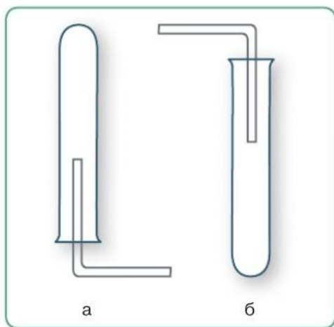
Рис. 61. Собираение газов методом вытеснения воздуха: а — если M газа меньше 29; б — если M газа больше 29
