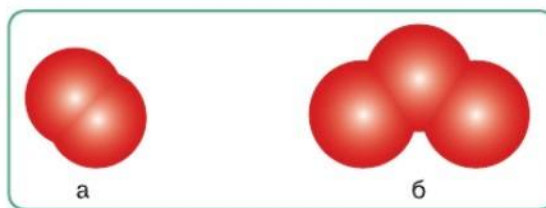
Рис. 29. Модели молекул аллотропных модификаций кислорода: а — кислород; б — озон
