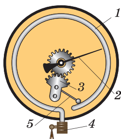
Рис. 144. Устройство металлического манометра
