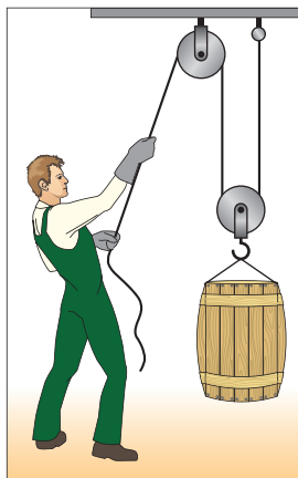
Рис. 185. Комбинация подвижного и неподвижного блоков — полиспаст
