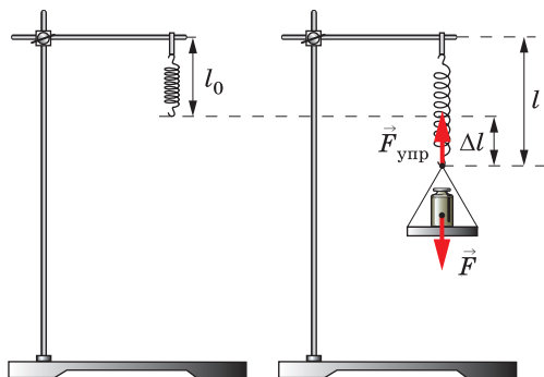
Рис. 71. Возникновение силы упругости при деформации
