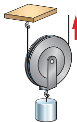
Рис. 183. Подвижный блок
