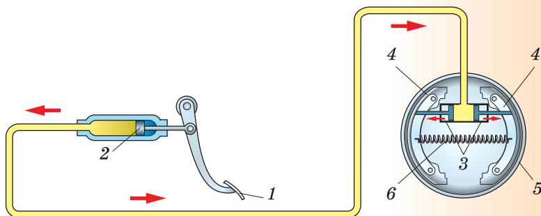
Рис. 150. Схема автомобильного гидравлического тормоза
