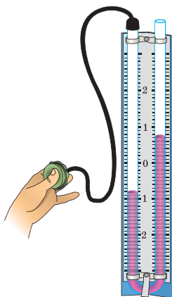
Рис. 141. Изменение уровня жидкости в коленях манометра
