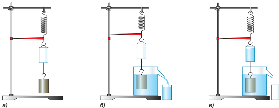
Рис. 154. Опыты с ведром Архимеда
