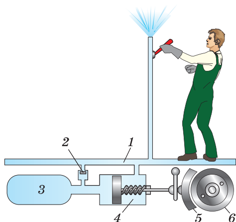
Рис. 109. Устройство пневматического тормоза
