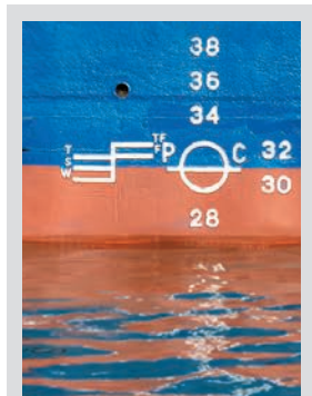
Отметки, определяющие грузовые ватерлинии судна при его загрузке в различных зонах, районах и в сезонные периоды плавания
