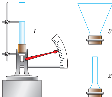
Рис. 118. Экспериментальная проверка гидростатического парадокса
