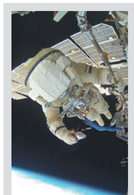
Состояние невесомости в космосе
