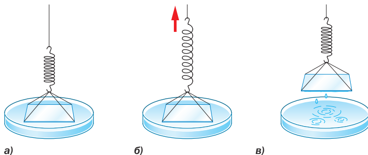
Рис. 30. Притяжение между молекулами стекла и воды
