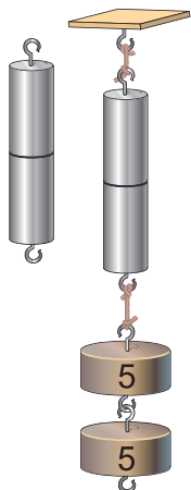
Рис. 29. Сцепление свинцовых цилиндров
