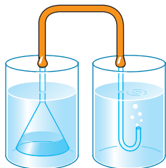
Рис. 32. Обнаружение воздуха в окружающем пространстве
