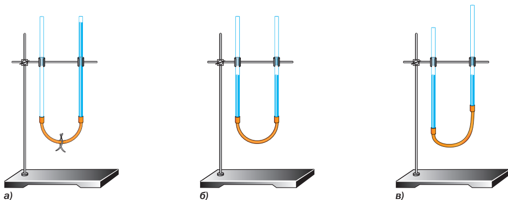
Рис. 119. Установление уровня жидкости в сообщающихся сосудах
