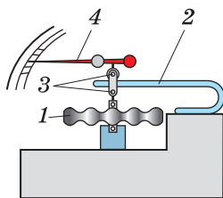
Рис. 138. Устройство барометра-анероида
