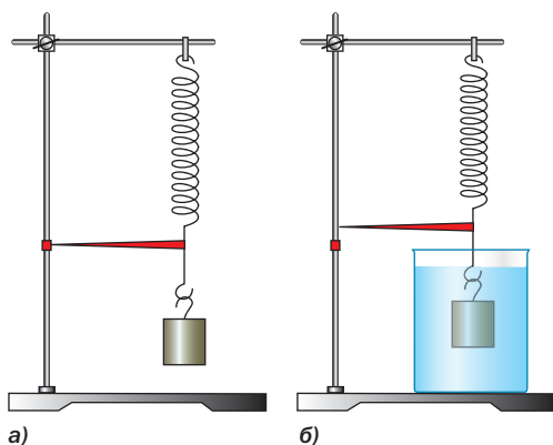
Рис. 152. Обнаружение силы, выталкивающей тело из жидкости
