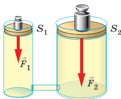
Рис. 147. Принцип действия гидравлической машины
