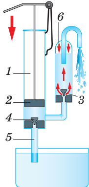
Рис. 146. Поршневой жидкостный насос с воздушной камерой
