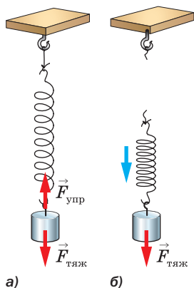
Рис. 74. После перерезания нити деформация пружины исчезает
