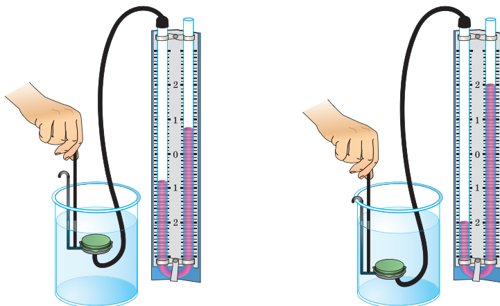
Рис. 142. Измерение давления жидкостным манометром
