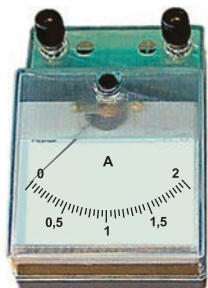
Рис. 9. Амперметр
