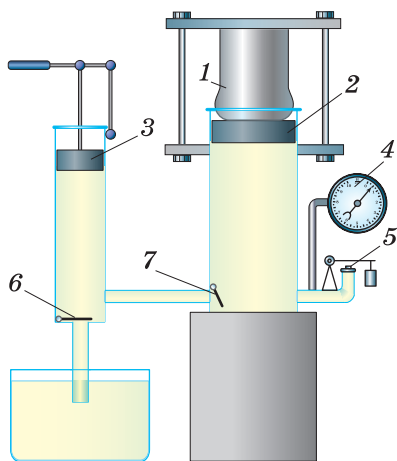
Рис. 148. Устройство гидравлического пресса
