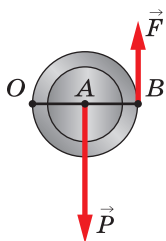
Рис. 184. Подвижный блок как рычаг с неравными плечами
