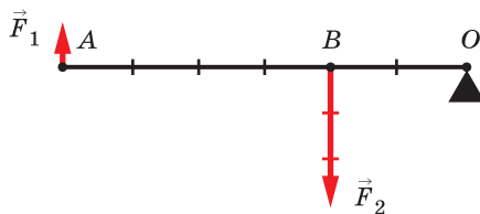
Рис. 172. Равновесие рычага второго рода
