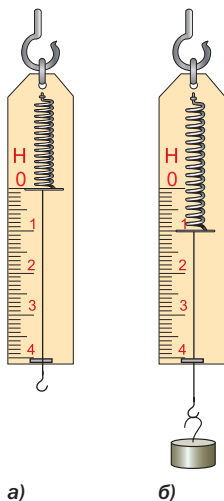
Рис. 77. Принцип действия динамометра
