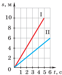
Рис. 40. График I соответствует телу, движущемуся с большей скоростью: v_I > v_{II}
