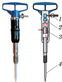
Рис. 108. Внешний вид и устройство пневматического отбойного молотка
