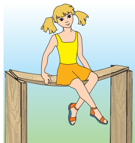
Рис. 62. Прогибание доски под действием тела человека
