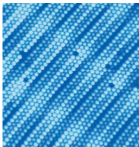
Рис. 24. Изображение атомов платины, полученное на туннельном микроскопе 1
