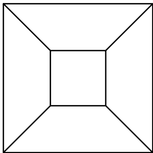
Рис. 98. Усечённая пирамида
