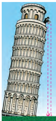
Рис. 1.6. Опыт Галилея
