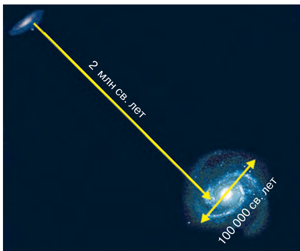
Рис. 4.11. Расстояния в мире галактик
