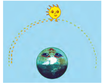
Рис. 4.9. Видимое движение Солнца
