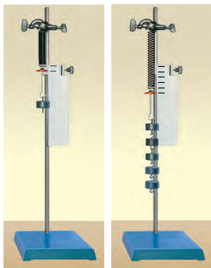
Рис. 12.4. Градуировка модели динамометра
