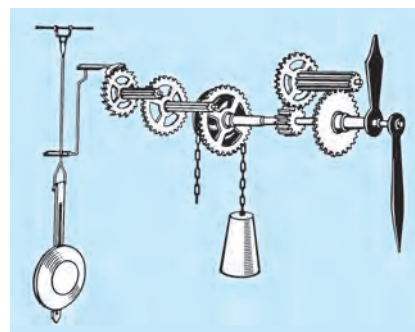
Рис. 3.6. Маятниковые часы
