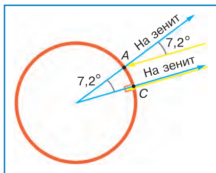
Рис. 2.5. Измерение радиуса Земли
