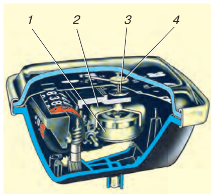
Рис. 6.4. Устройство автомобильного спидометра
